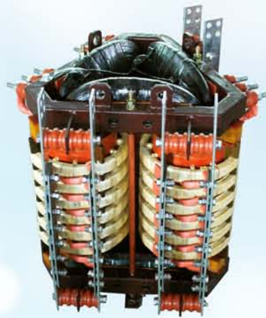
▼ 自耦变压器-低压
