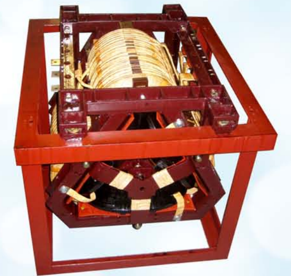
▼ 电力机车用辅助变压器
